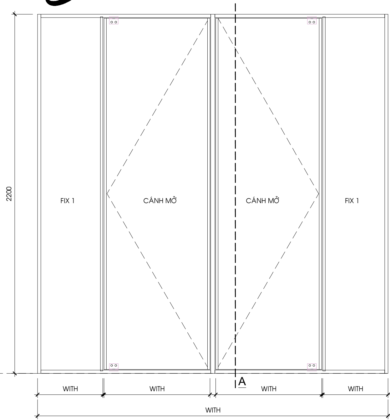
MẶT ĐỨNG
